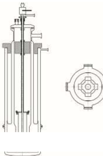
Криостат для оптических измерений и съемный держатель образца
