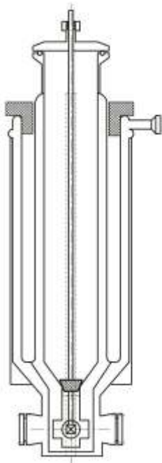
Криостат для оптических измерений
