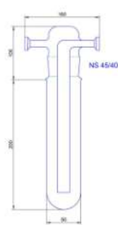
Typ S 29-NW16-Z / NW25-Z
